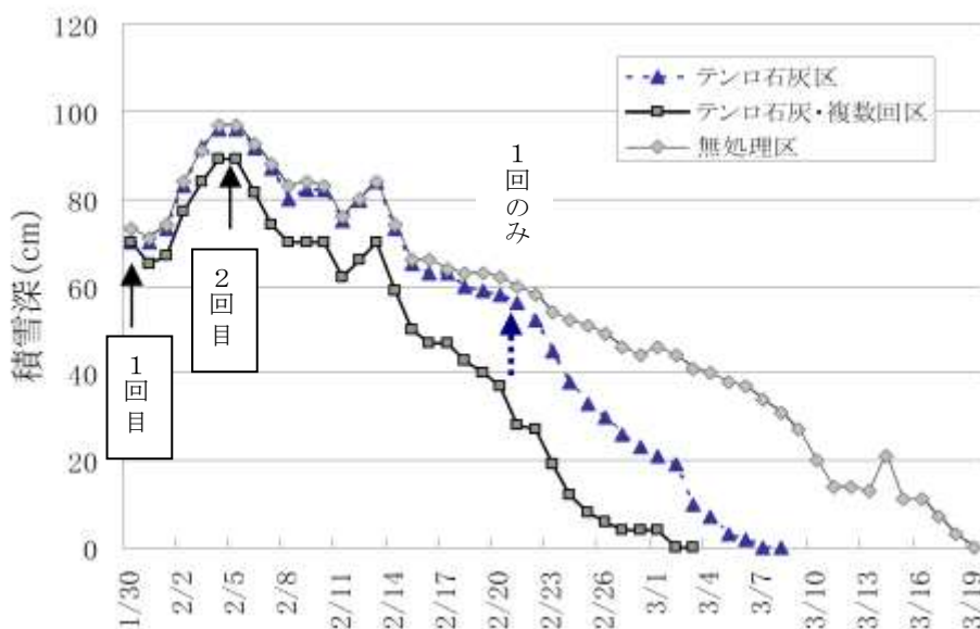
図2 融雪剤の散布時期、回数の違いと消雪効果 (農業総合研究センター園芸試験場 平成18年)
